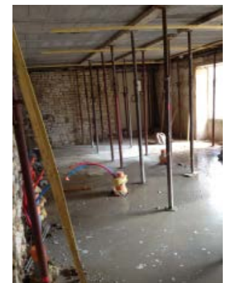
Dalles de béton pour le rez-de-chaussée et l'étage
